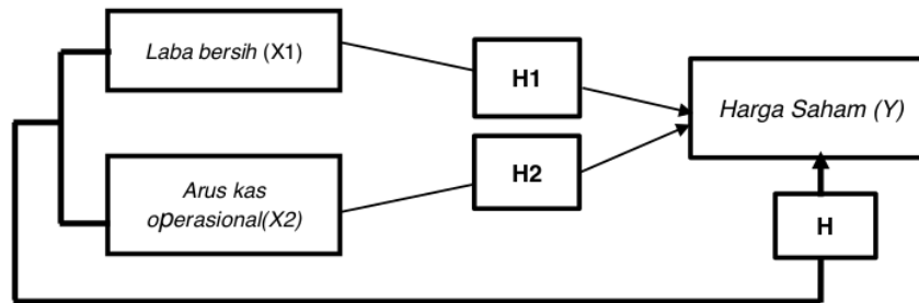
Gambar 1. Kerangka Berpikir
