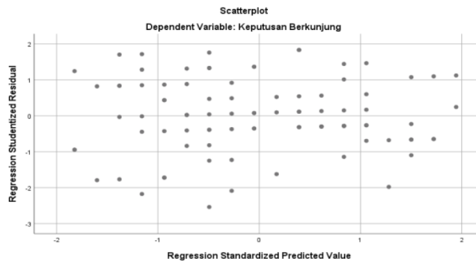
Gambar 2 Uji Heteroskedastisitas Scatteplot
