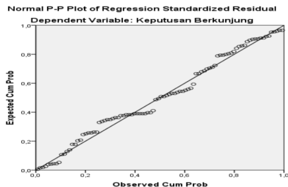
Gambar 1 Uji Normalitas
