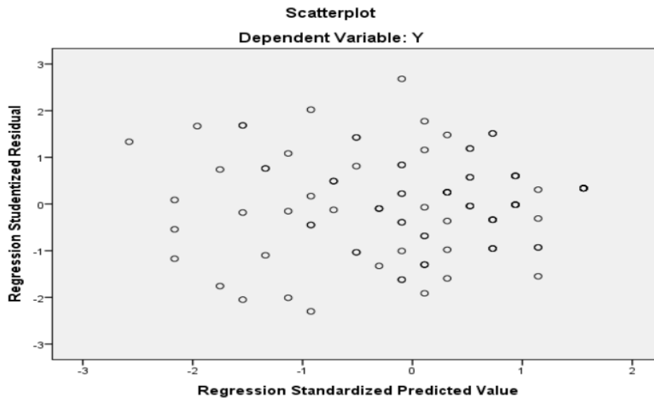
Gambar 2 Uji Heteroskedastisitas Scatterplot
